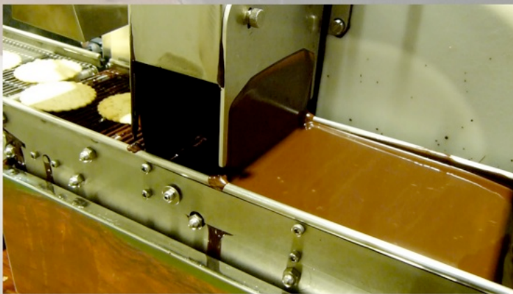
全面エンロービングの場合に 製品が出来るだけ長い区間 チョコレートに浸かれるような デザインになっています。
