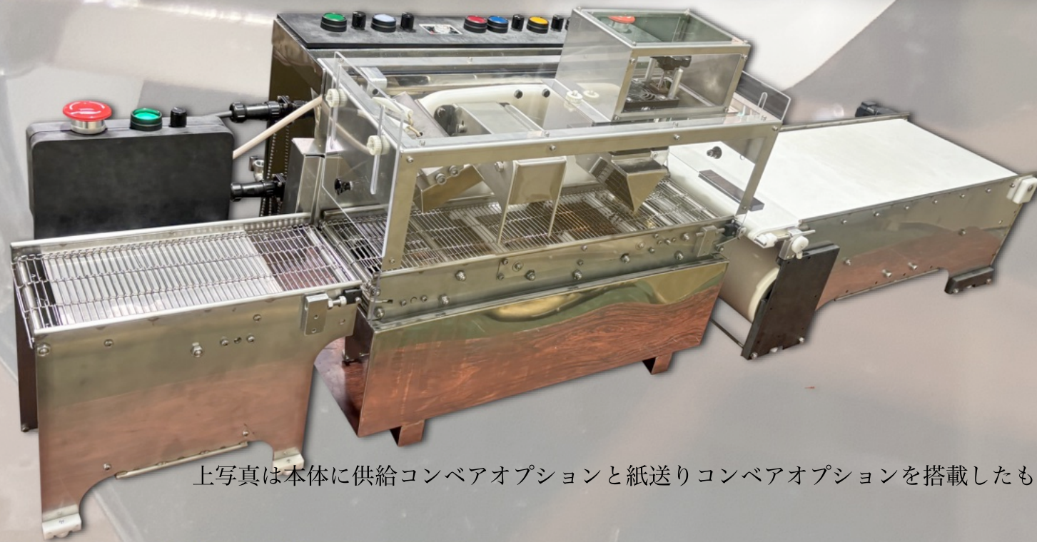
全面エンロービングの場合に 製品が出来るだけ長い区間 チョコレートに浸かれるような デザインになっています。
